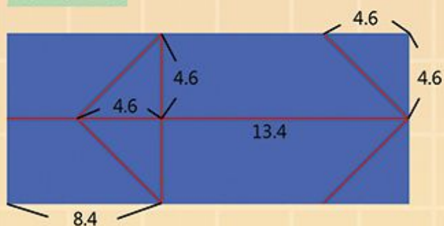
紙A示意圖 9.2x21.8 cm
